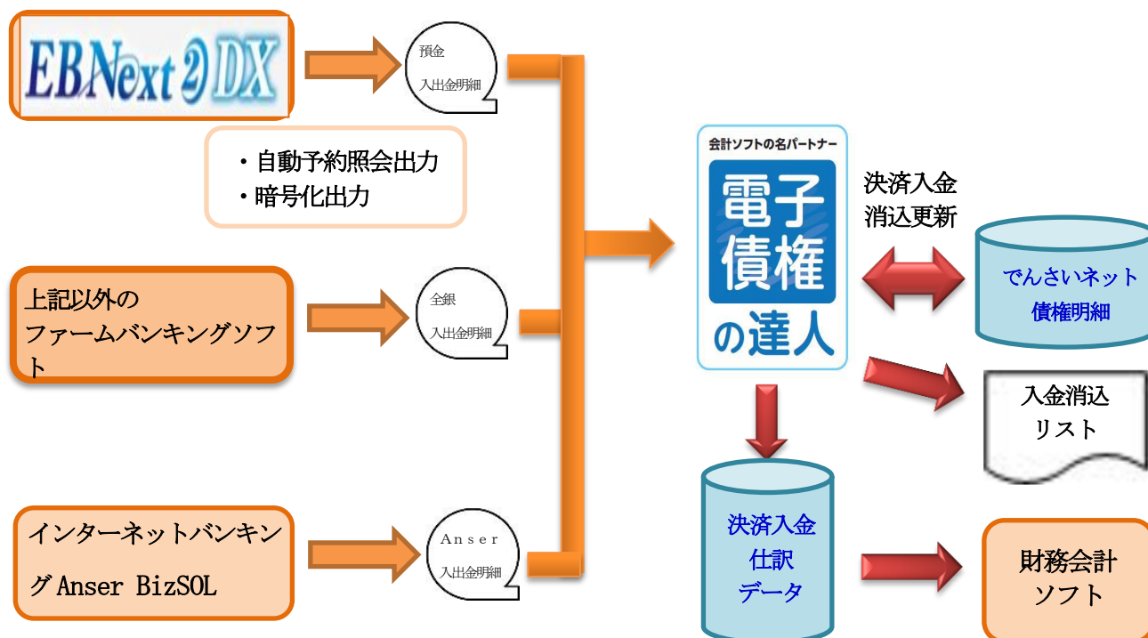
1-1 決済入金即日消込機能 概要図
